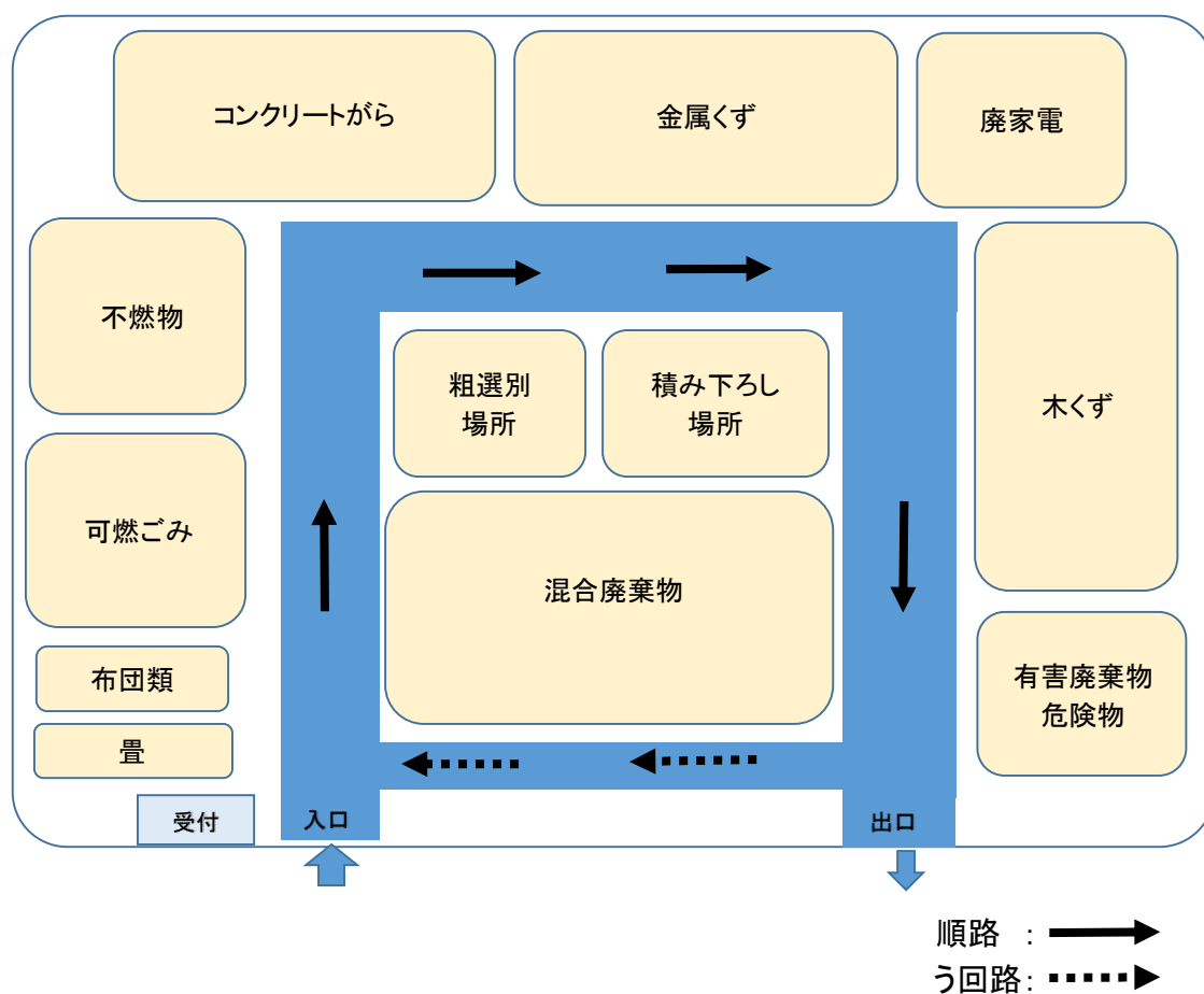
図４－３ 仮置場のレイアウト例
