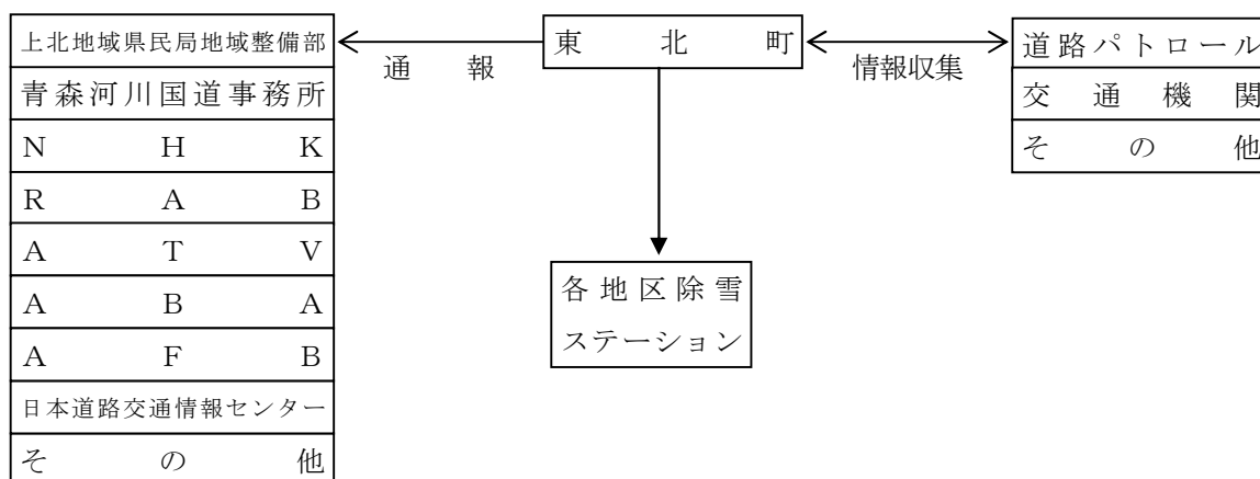
豪雪時における連絡系統図
